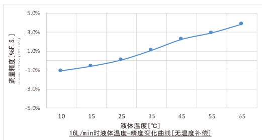
使用产品：FML-303 对比液温 25°C 测量结果所产生的偏差 [%FS]
